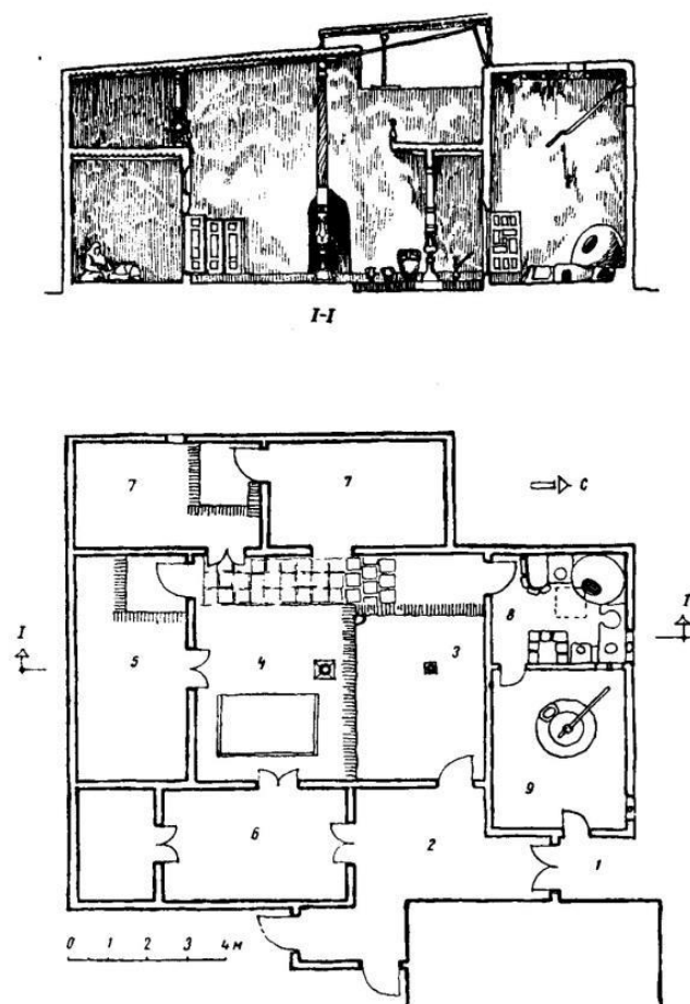
2-расм. Хивадаги Якуббо хўжа турар уй-жойи XIX-аср охири 1-кириш; 2-дахлиз; 3-терс айвон; 4-улли айвон; 5-сарой; 6-пеш уй; 7- ёнбош уй; 8- ошхона; 9-хорозхона
