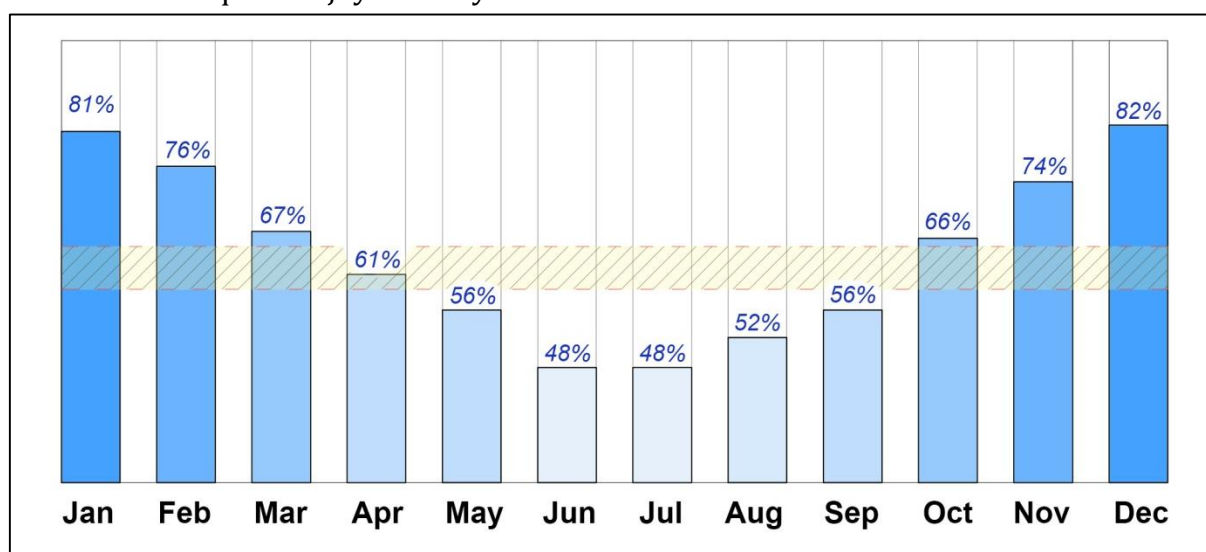
1- rasm. Farg'ona viloyati havo namligi sharoitlarini baholash
