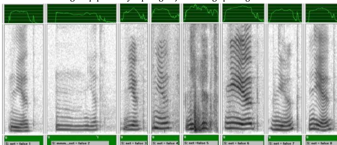
2-rasm: So'zlovchining yolg'ondan "yo'q" degan javobining spektogrammasi.
