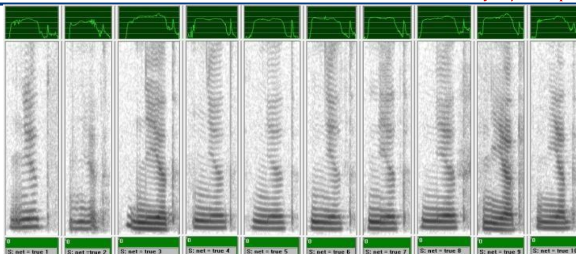
1-rasm: So'zlovchining haqiqatdan "yo'q" degan javobining spektogrammasi.
